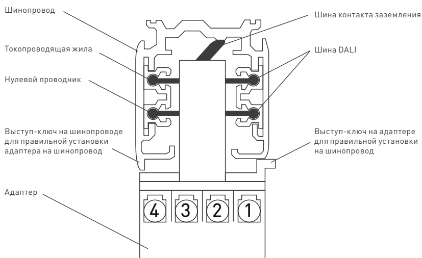
Рис. 1. Подключение адаптера к шинопроводу
