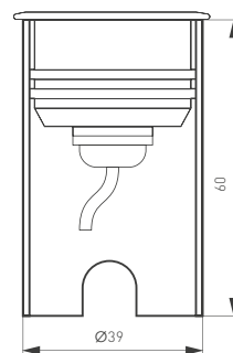
Рис.2. Чертеж и габаритные размеры монтажной втулки
