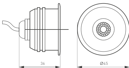
Рис.1. Чертеж и габаритные размеры светильника
