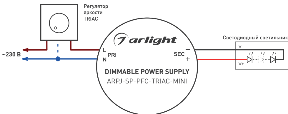
Рис. 1. Подключение драйвера.
