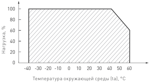
Рис. 2. Максимальная допустимая нагрузка, % от мощности источника
