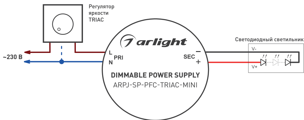
Рис. 1. Подключение драйвера.
